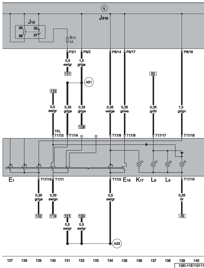
大灯旋转开关, 后雾灯
